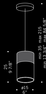
CONCERTO S35 1x35W G12 scarica metal halide high intensity discharge alimentatore elettronico electronic ballast
